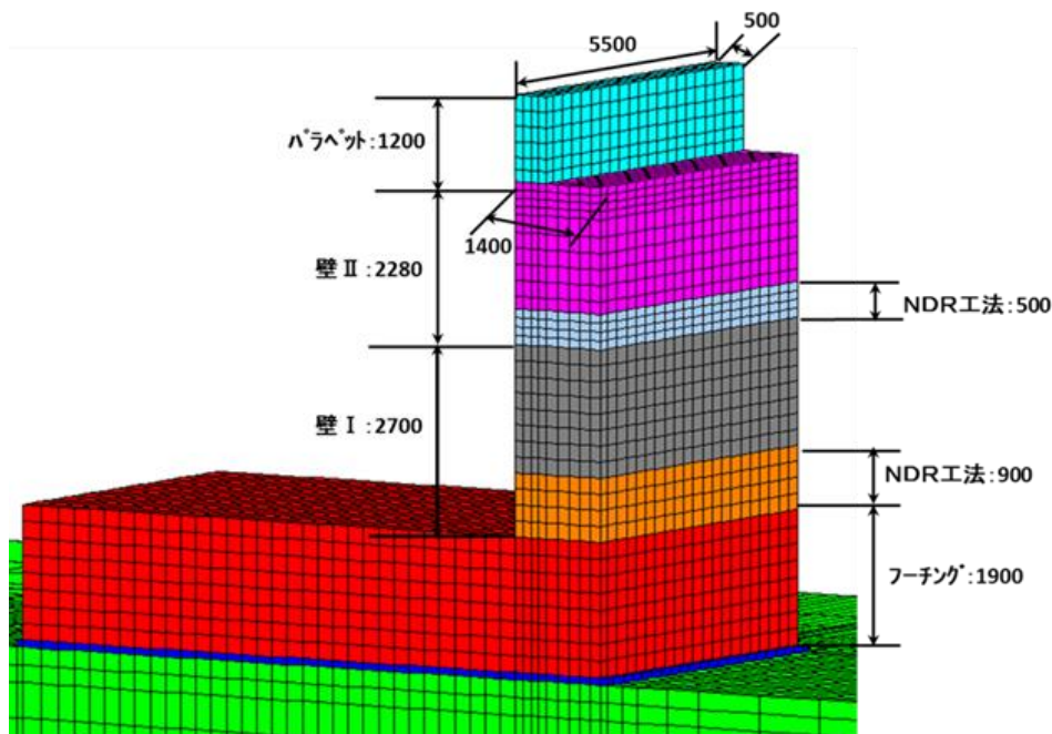
解析: 1/2対象モデル
