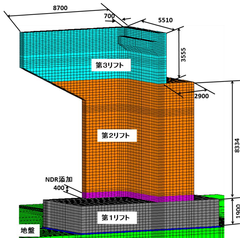
解析: 1/2対象モデル
