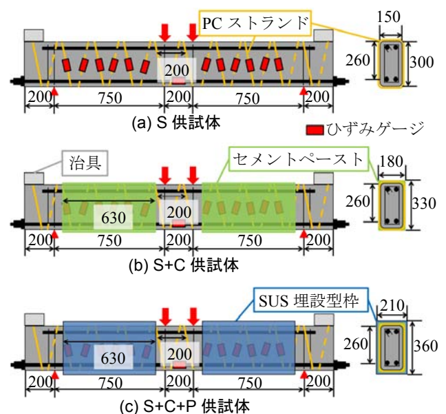
図 1 RC はり供試体図(単位: mm)
