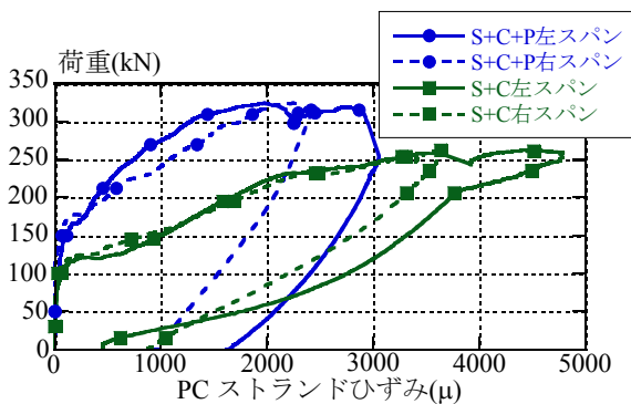
図 5 荷重—PC ストランドひずみ関係
