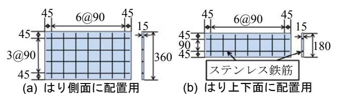
図 2 SUS 埋設型枠図(単位: mm)
