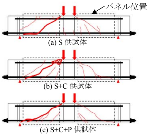
図 4 ひび割れ状況(太線は顕著なもの、斜線部はコンクリート圧壊部分)
