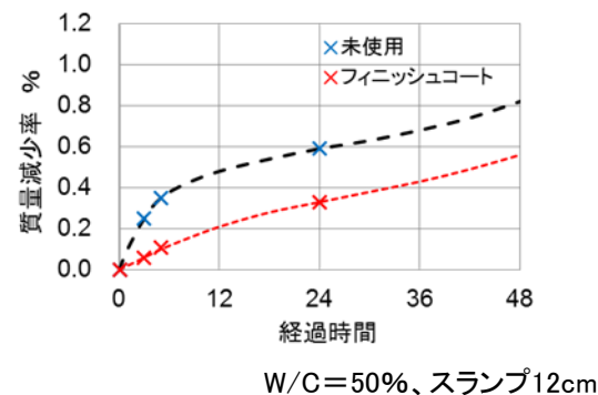
コンクリート表面からの水分逸散量試験結果
